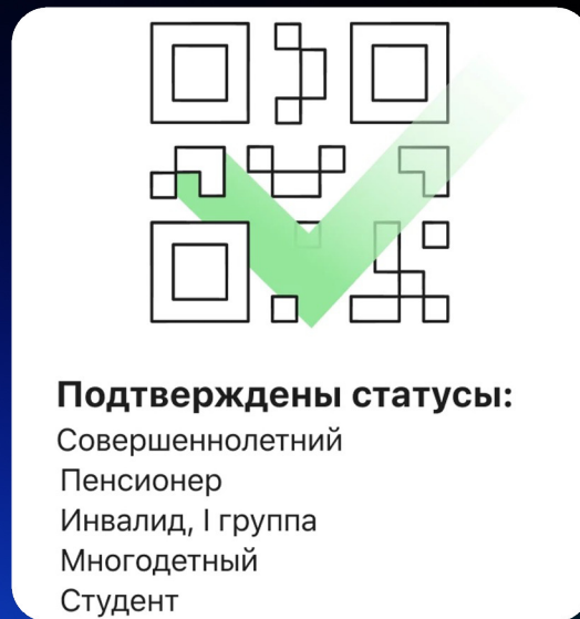
Кассовое ПО
